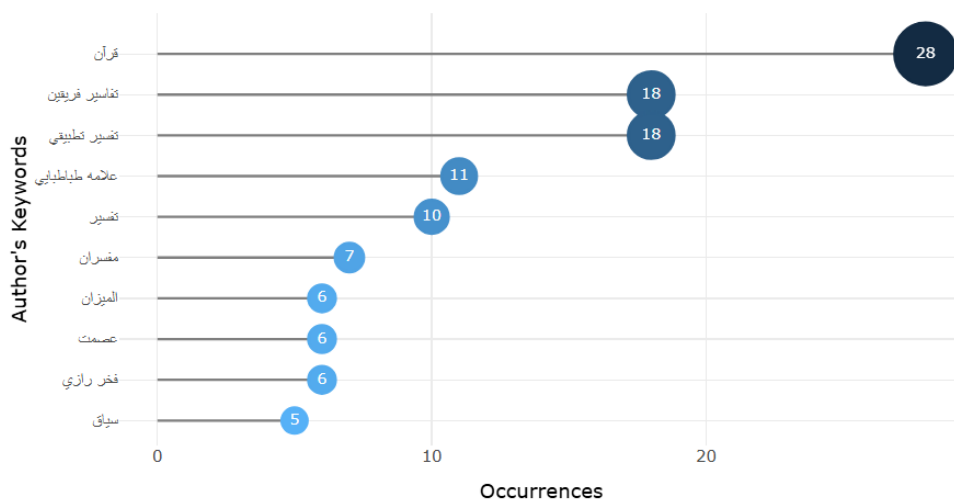
شکل ۴. پرسامدترین کلیدواژه‌ها
